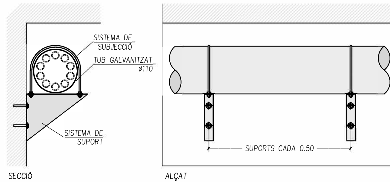
DETALL - A
