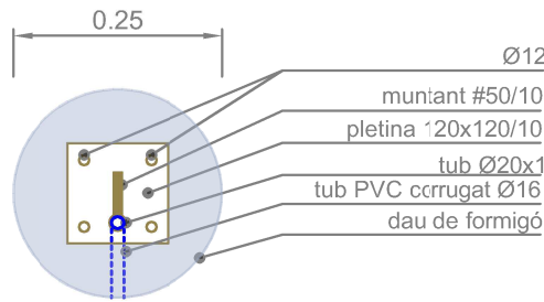
ANCLATGE AMB TUB PER A ALIMENTACIÓ DE INSTAL·LACIÓ LEDS
