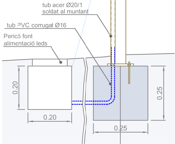
DETALL MUNTANT AMB ALIMENTACIÓ IL·LUMINACIÓ CONTINUA A PASSAMÀ
