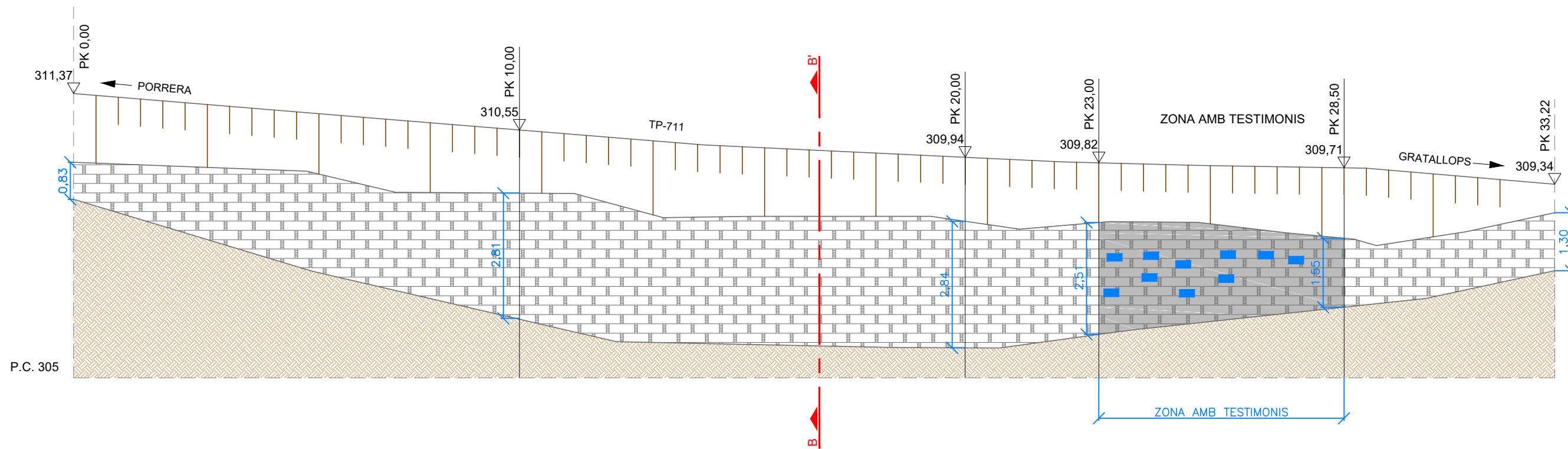
ALÇAT A-A' E:1/100
