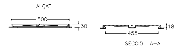
TAPA DE PERICÓ TIPUS "B" E 1/20
